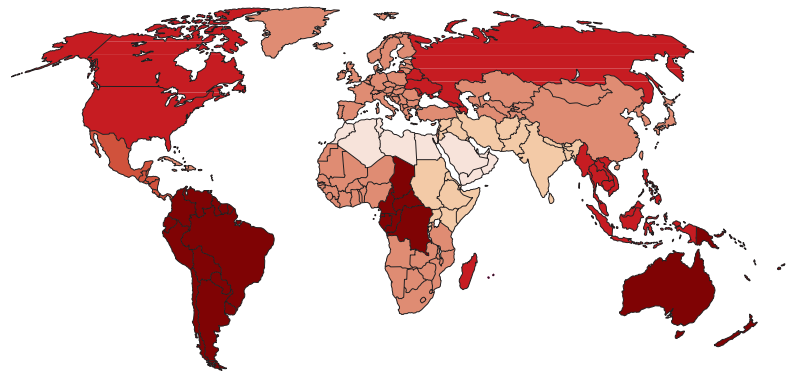
El mapa muestra la disponibilidad de agua medida en 1 000 m 3 /cápita/año.
