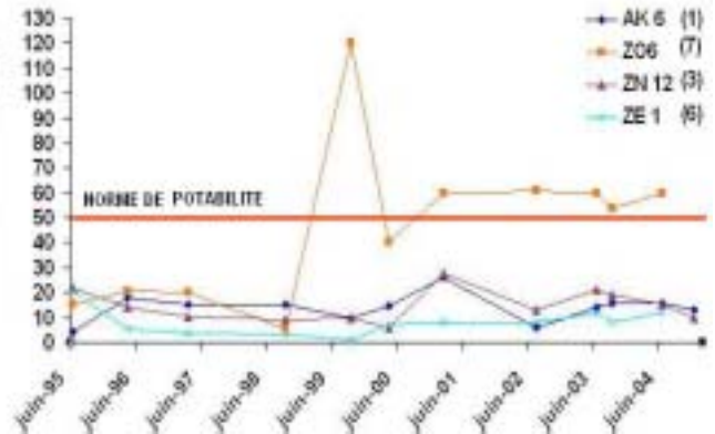
VARIATION DU TAUX DE NITRATES DANS QUELQUES FORAGES DE L'AQUIFERE D'ABIDJAN DE JUIN 95 A DECEMBRE 04
