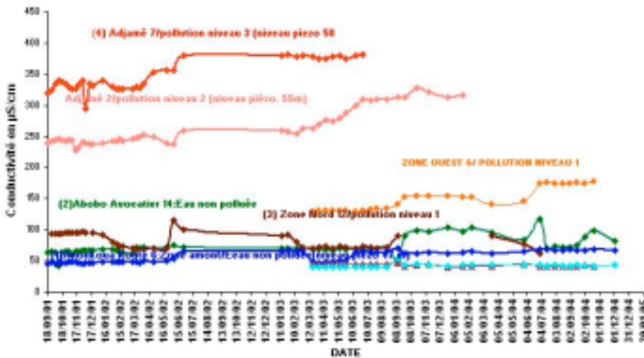
VARIATION DE LA CONDUCTIVITE DE L'AQUIFERE D'ABIDJAN DE SEPTEMBRE 2001 A DECEMBRE 2004
